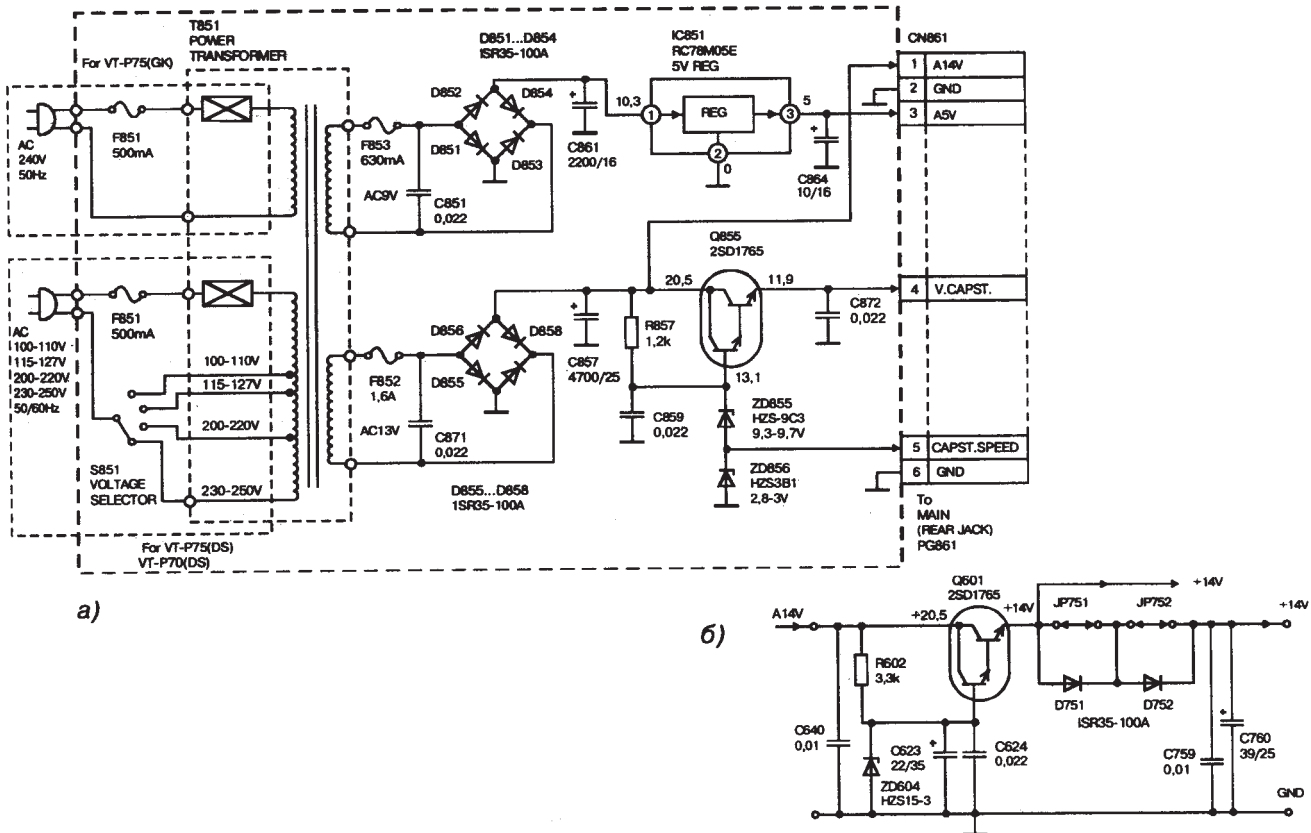
Принципиальная схема источника питания видеомэгнитофонов VT-P70/P75/P88 (а) и схема узла стабилизатора напряжения +14 В (б).
